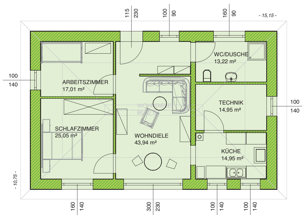
Erdgeschoss
